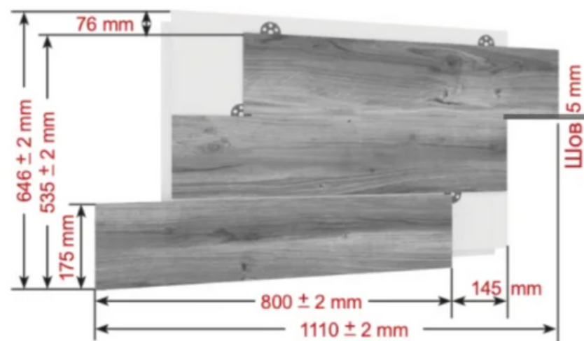
Прямой элемент 800/175
