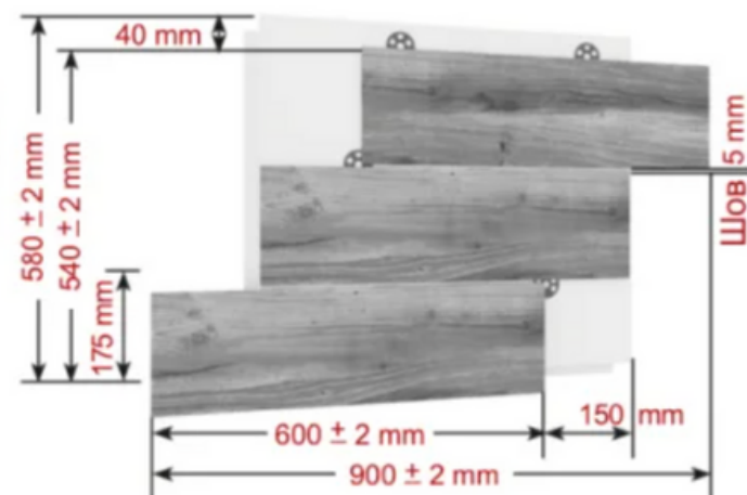
Прямой элемент 600/175
