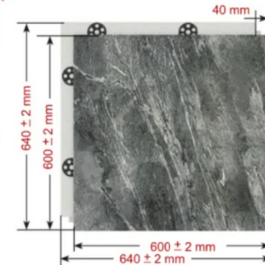
Прямой элемент 600/600
