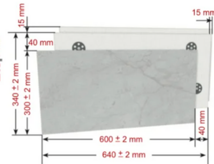
Прямой элемент 600/300
