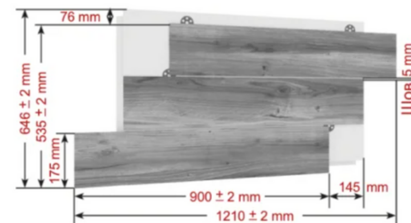
Прямой элемент 900/175
