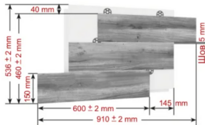
Прямой элемент 600/150
