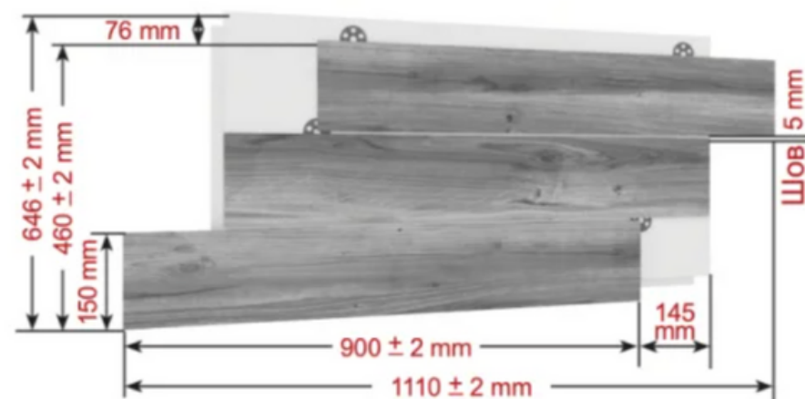
Прямой элемент 900/150
